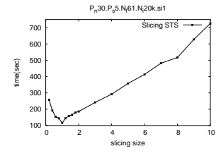
(d) Performance w.r.t Slicing Size
